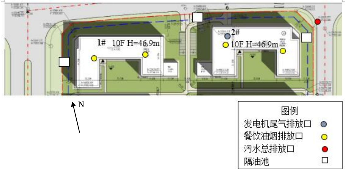
图3.3-3 建设项目平面布置图
